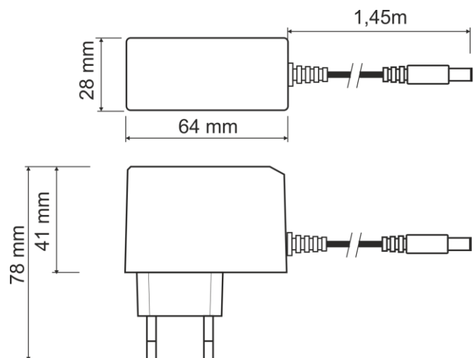
Rys.1. Widok mechaniczny zasilacza.
